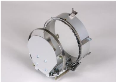
Kapfenstick-Einrichtung
